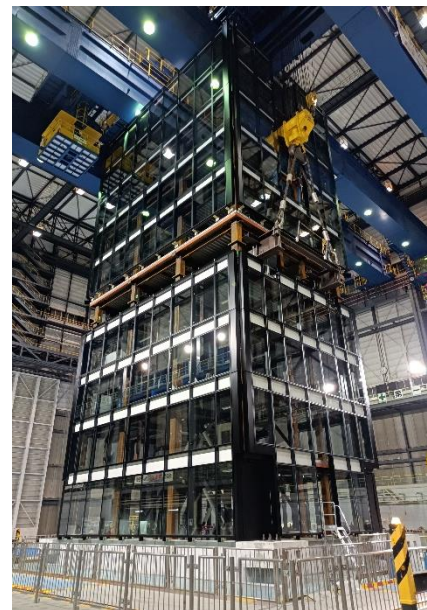
(b) 震動台への設置
